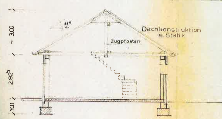
SCHNITT B-B
