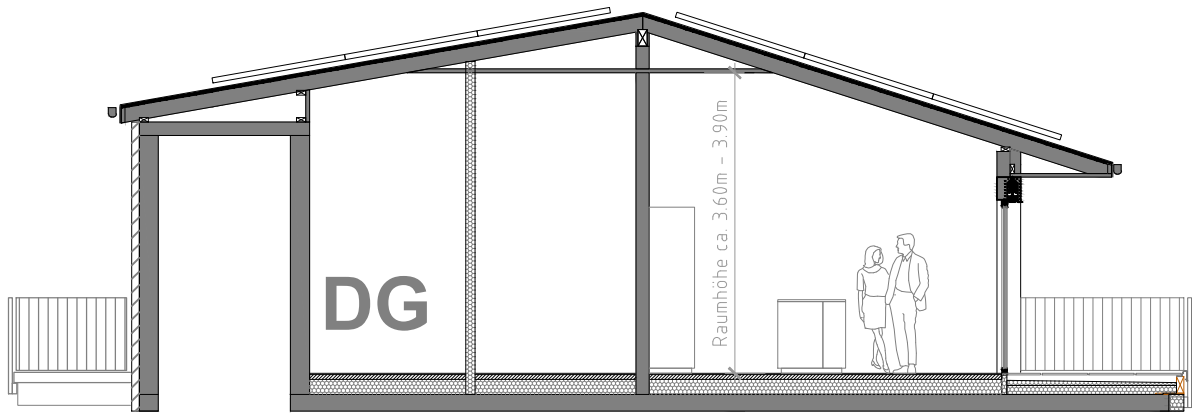
Schnitt A-A
