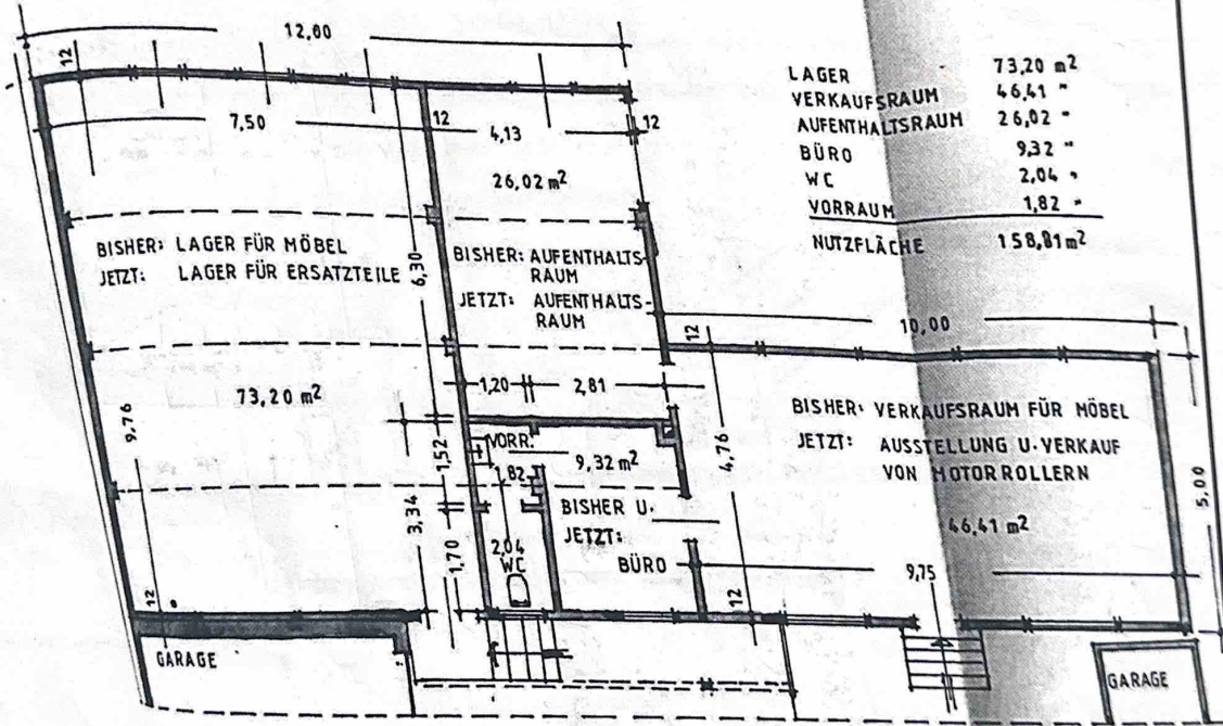
GRUNDRISS
