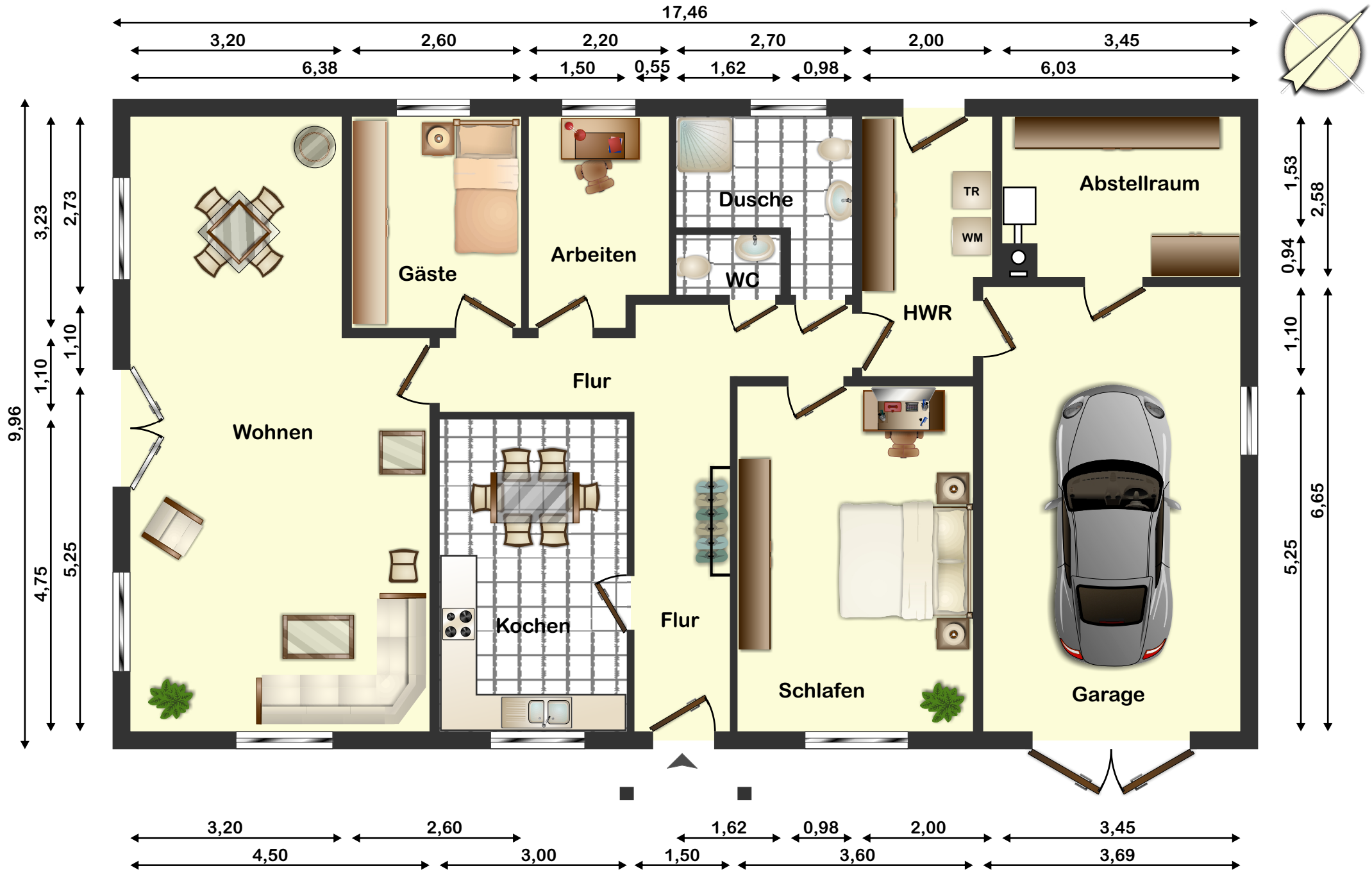
Erdgeschoss
