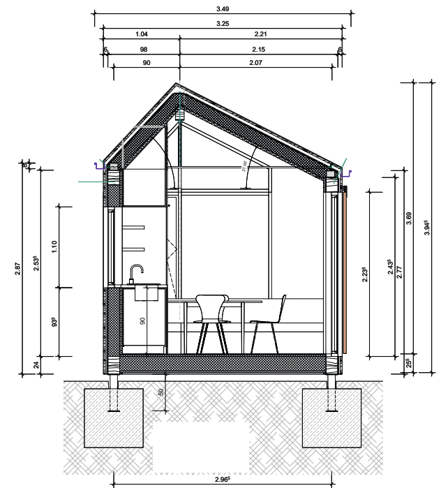
Querschnitt Küche
