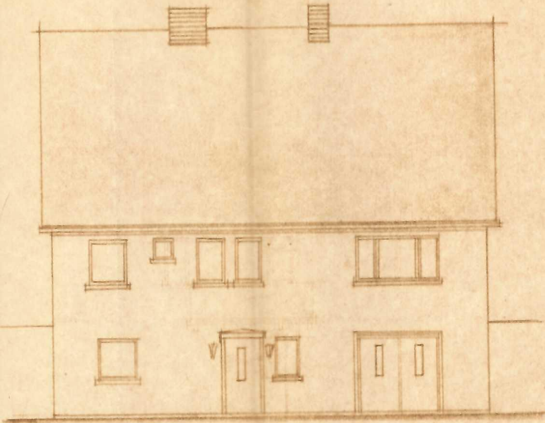
ANSICHT - NORD-OST.
