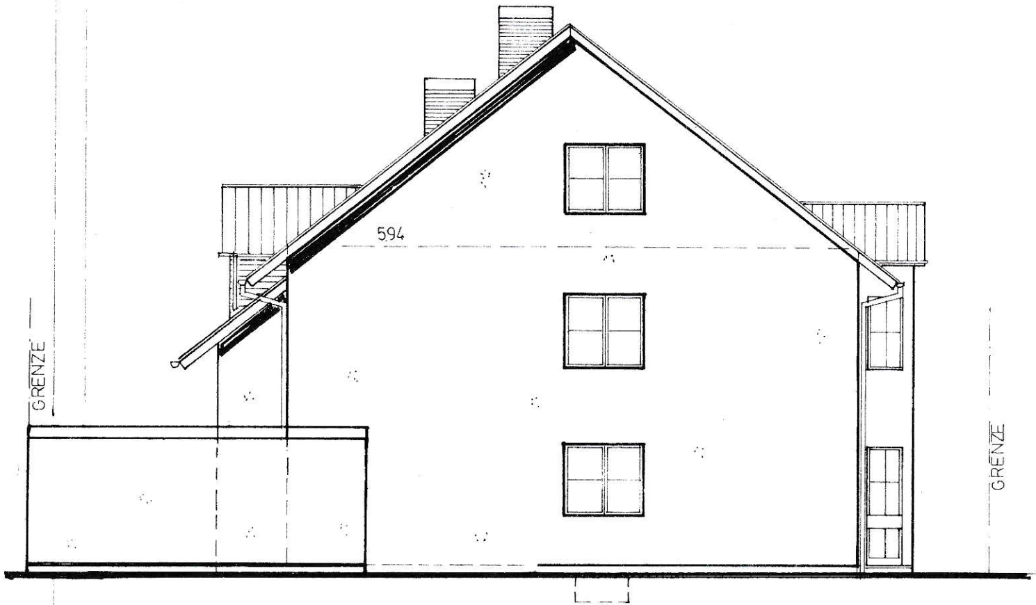
SÜDANSICHT
