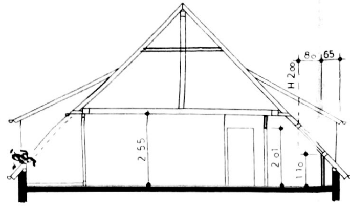
SCHNITT
