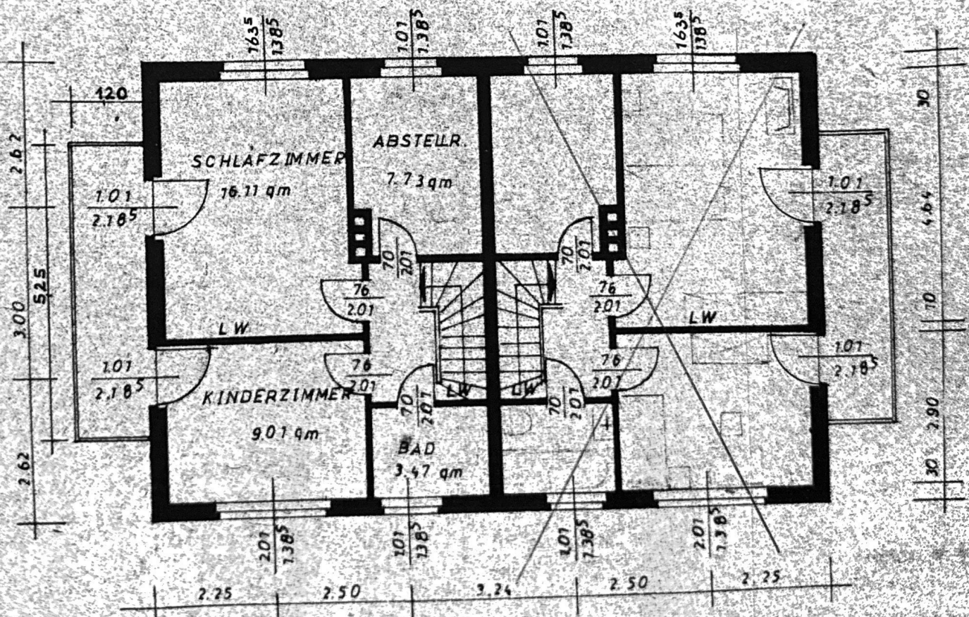
ERDGESCHOSS
