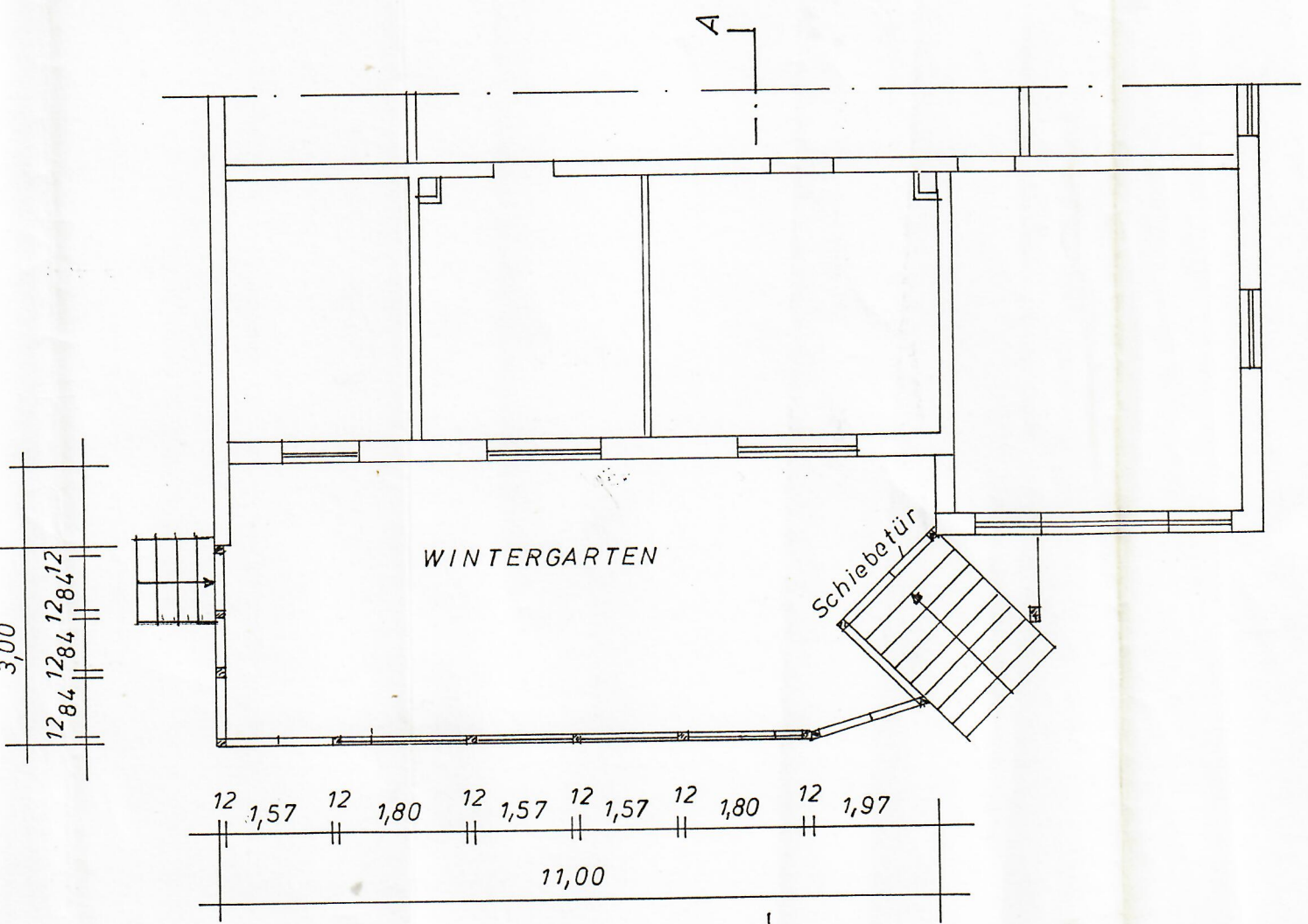
Grundriß
