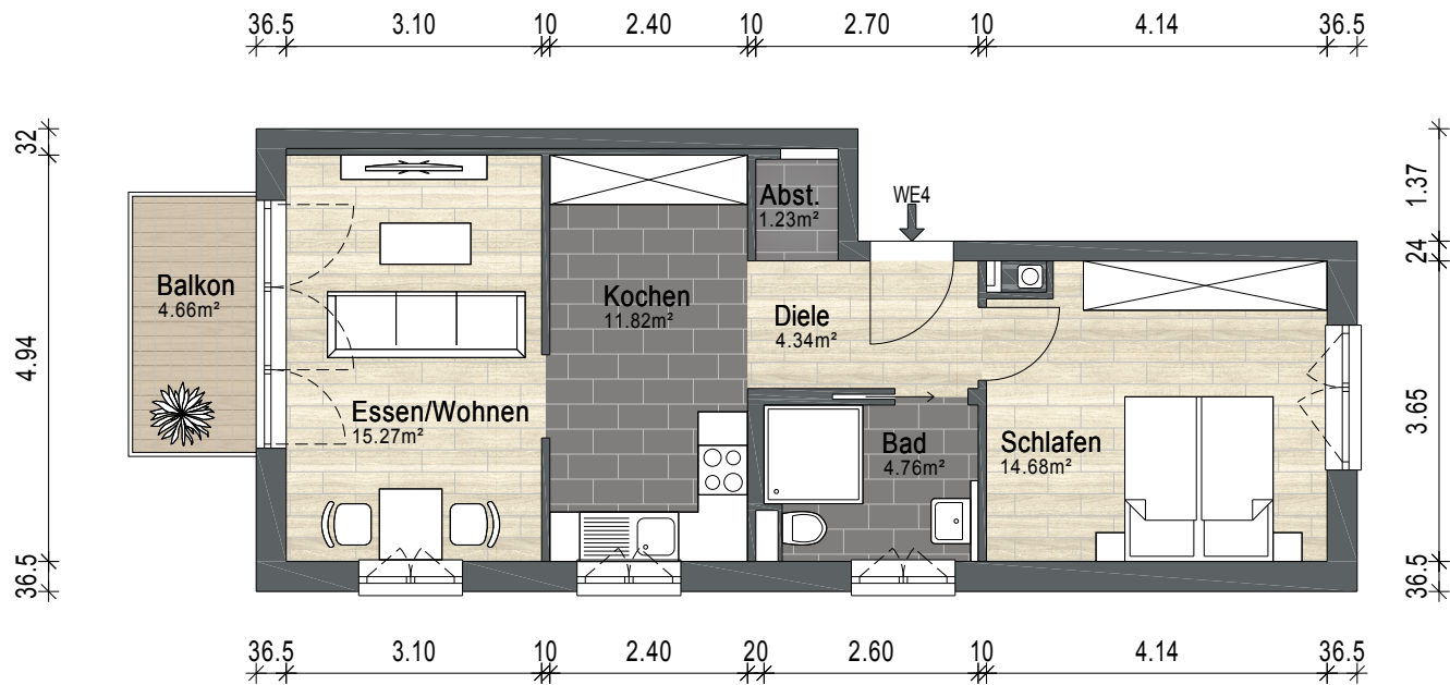
1.Obergeschoss
