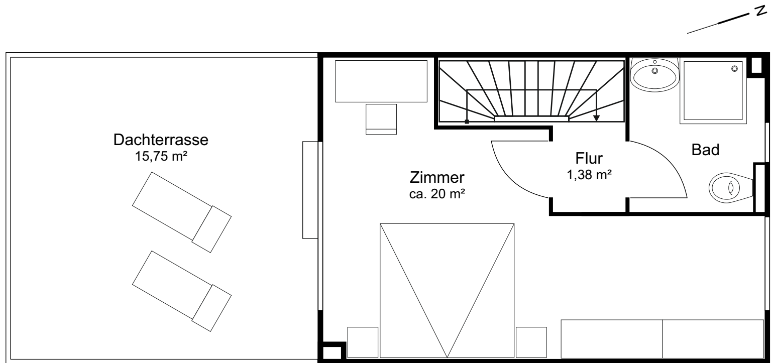
Staffelgeschoss
