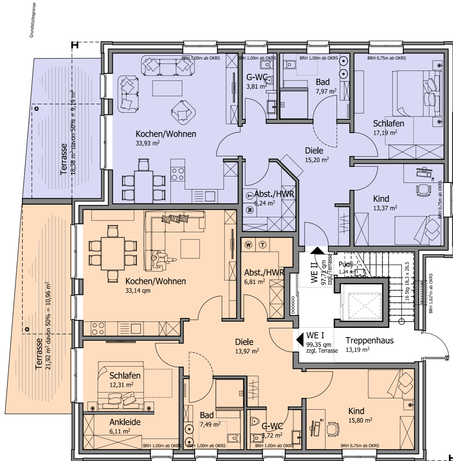
GRUNDRISS ERDGESCHOSS
