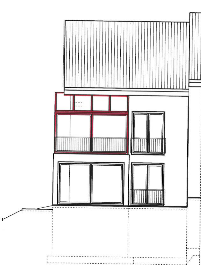
WESTANSICHT
