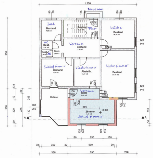
ERDGESCHOSS
