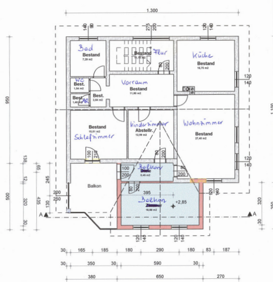
DACHGESCHOSS
