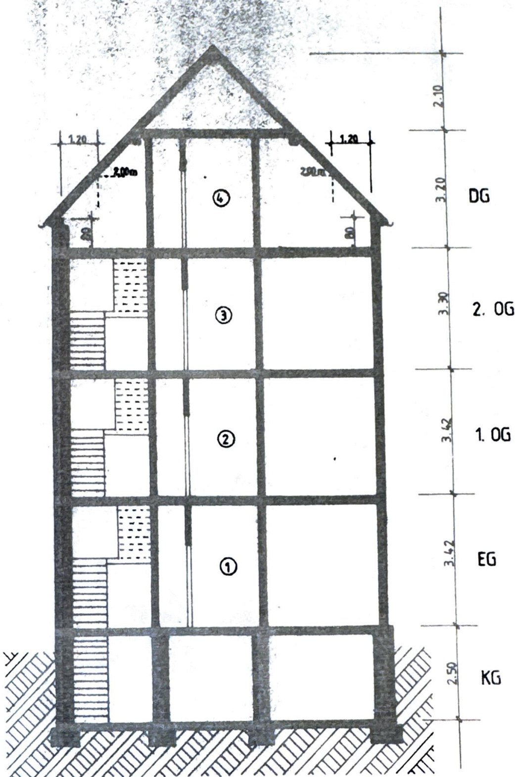
QUERSCHNITT
