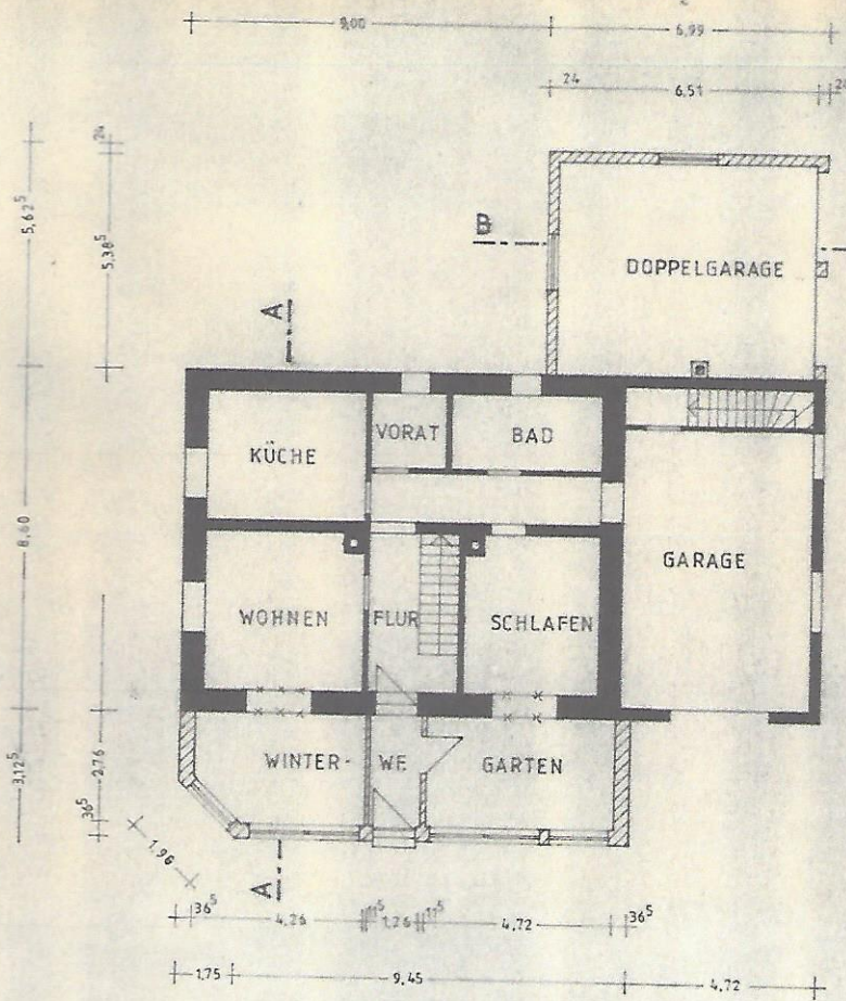
GRUNDRISS
