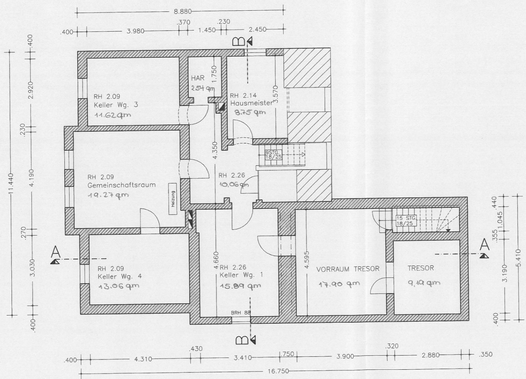
GRUNDRISS KELLERGESCHOSS
