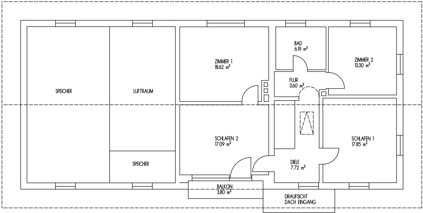
OBERGESCHOSS
