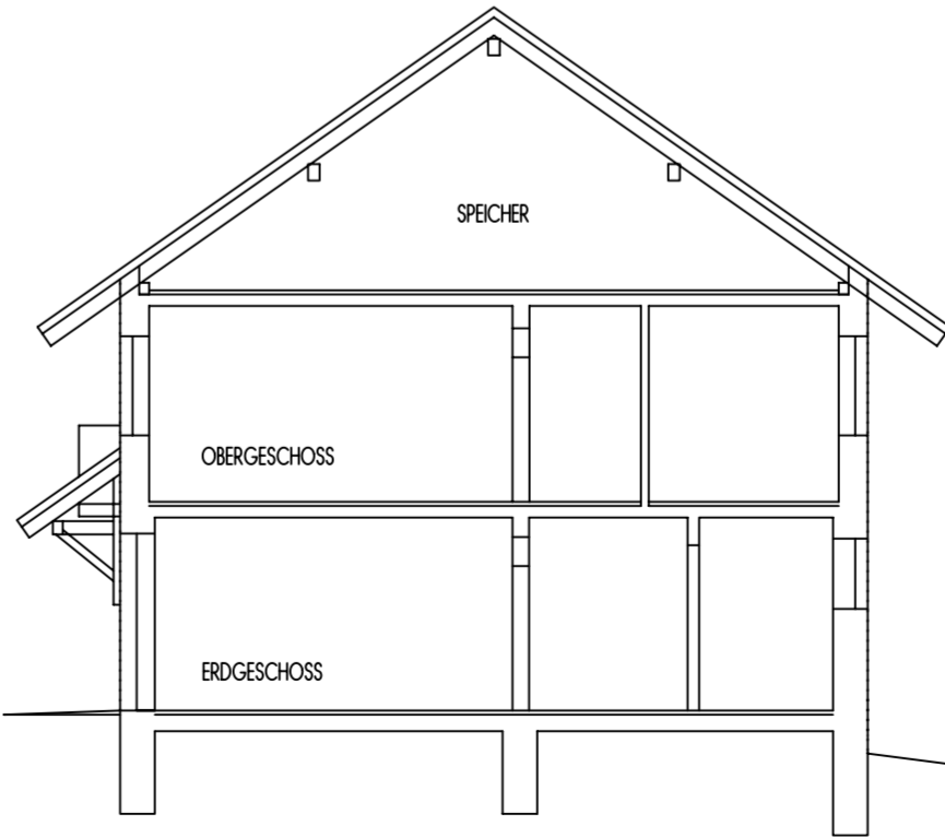
SCHNITT
