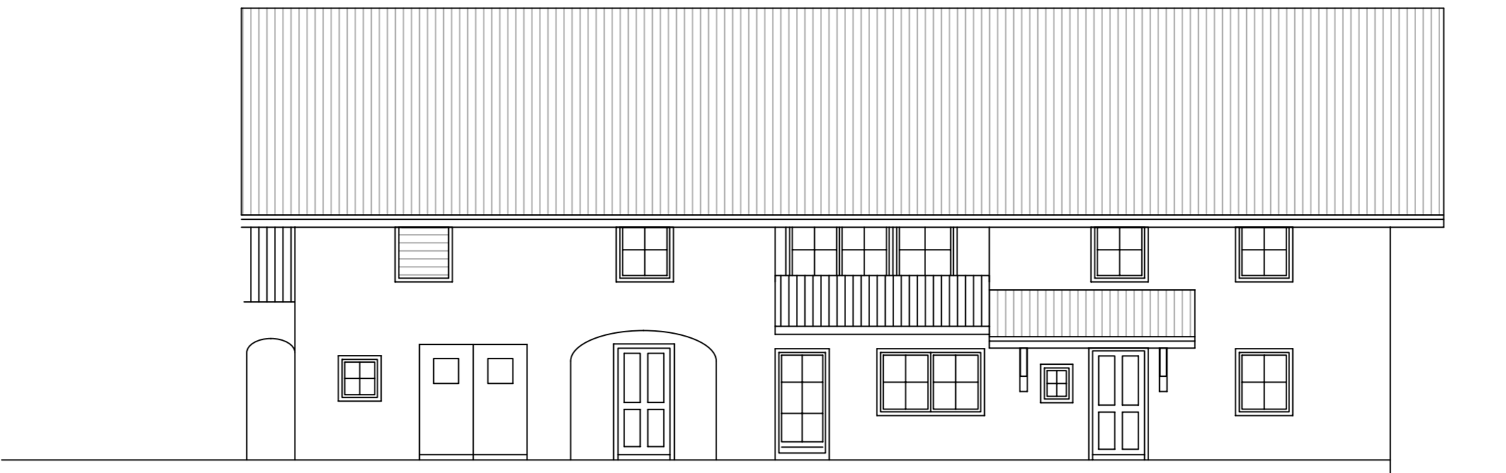
SUD-ANSICHT
