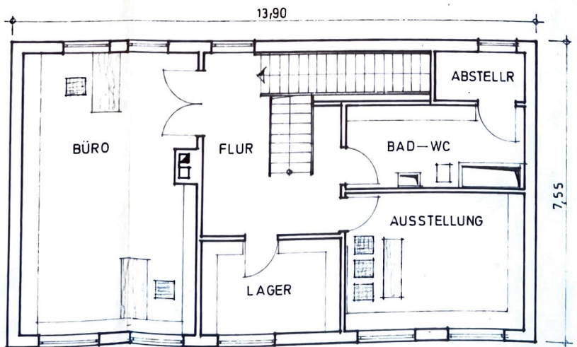
ERDGESCHOSS NACH DEM UMBAU
