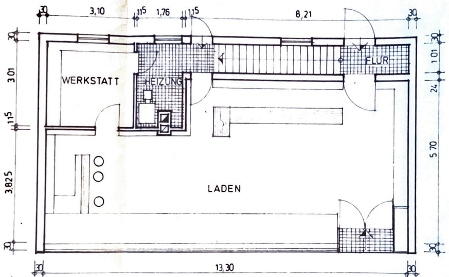
ERDGESCHOSS NACH DEM UMBAU
