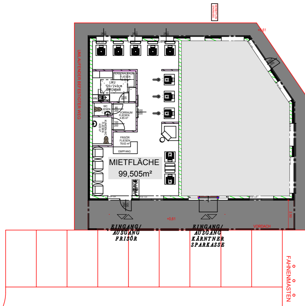
GRUNDRISS M 1:200
