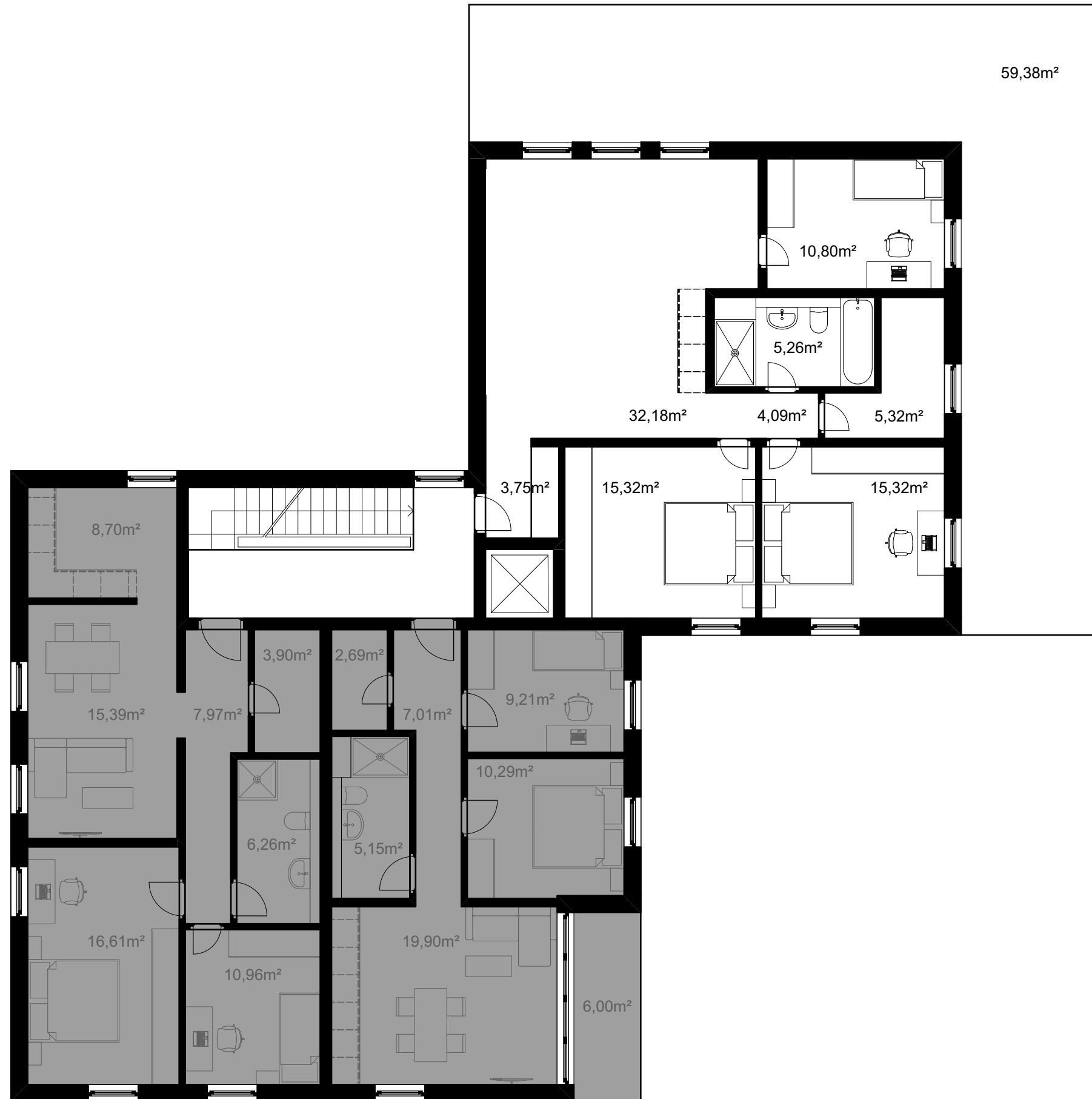
Grundriss 3. Obergeschoss
