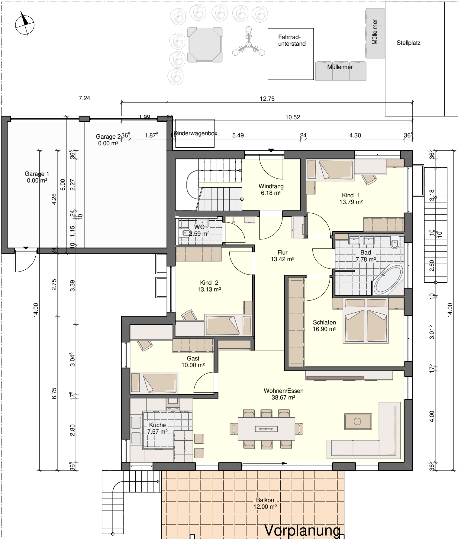
Dreifamilienhaus mit Doppelgarage Schönblickstraße 10 Winnenden-Breuningsweiler Erdgeschoss M 1:100
