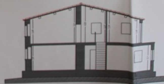
Sezione BB'
