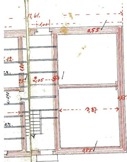
Kellergeschoß
