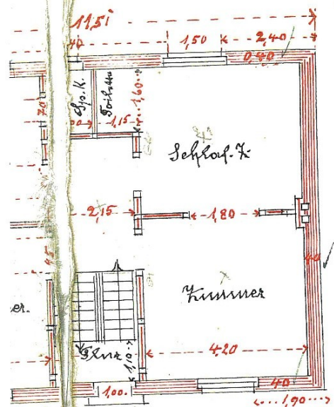
1. Geschoß
