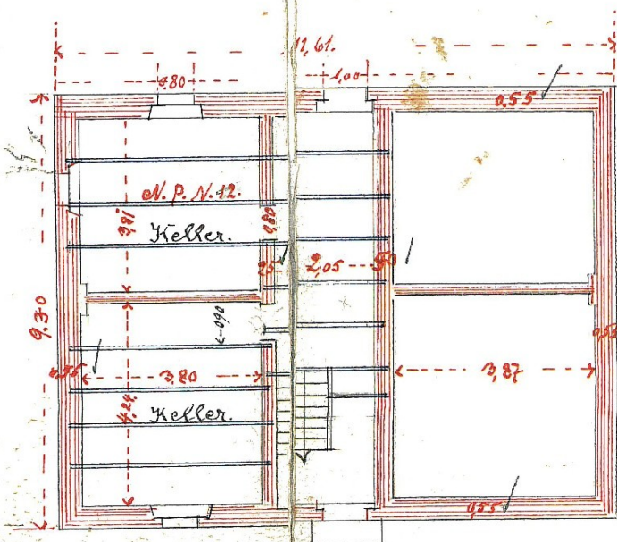
Keller
