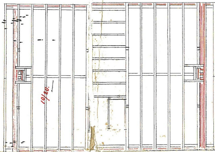
Dachstuhl Sparrenlage
