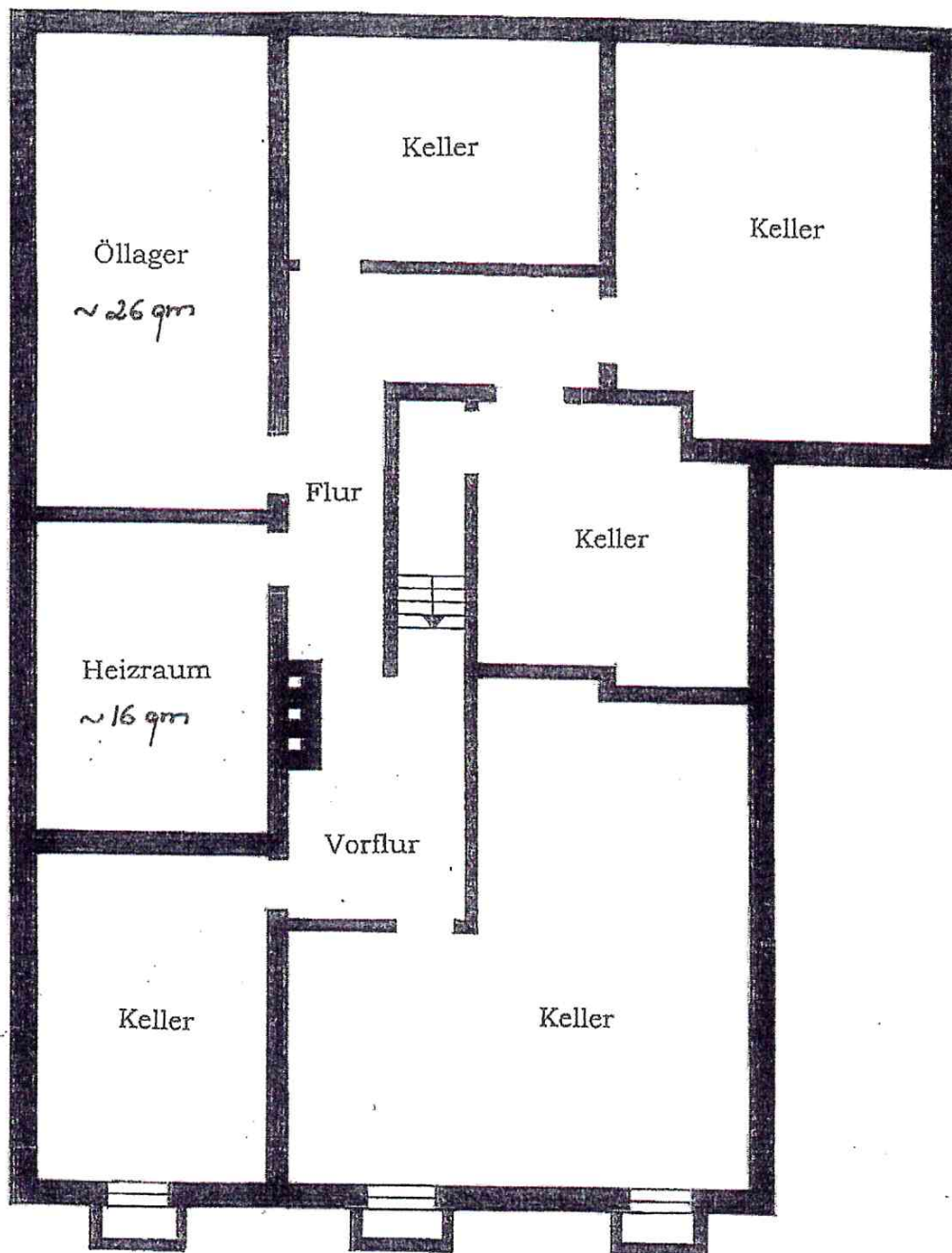
Kellergeschoss Maßstab 1 : 100
