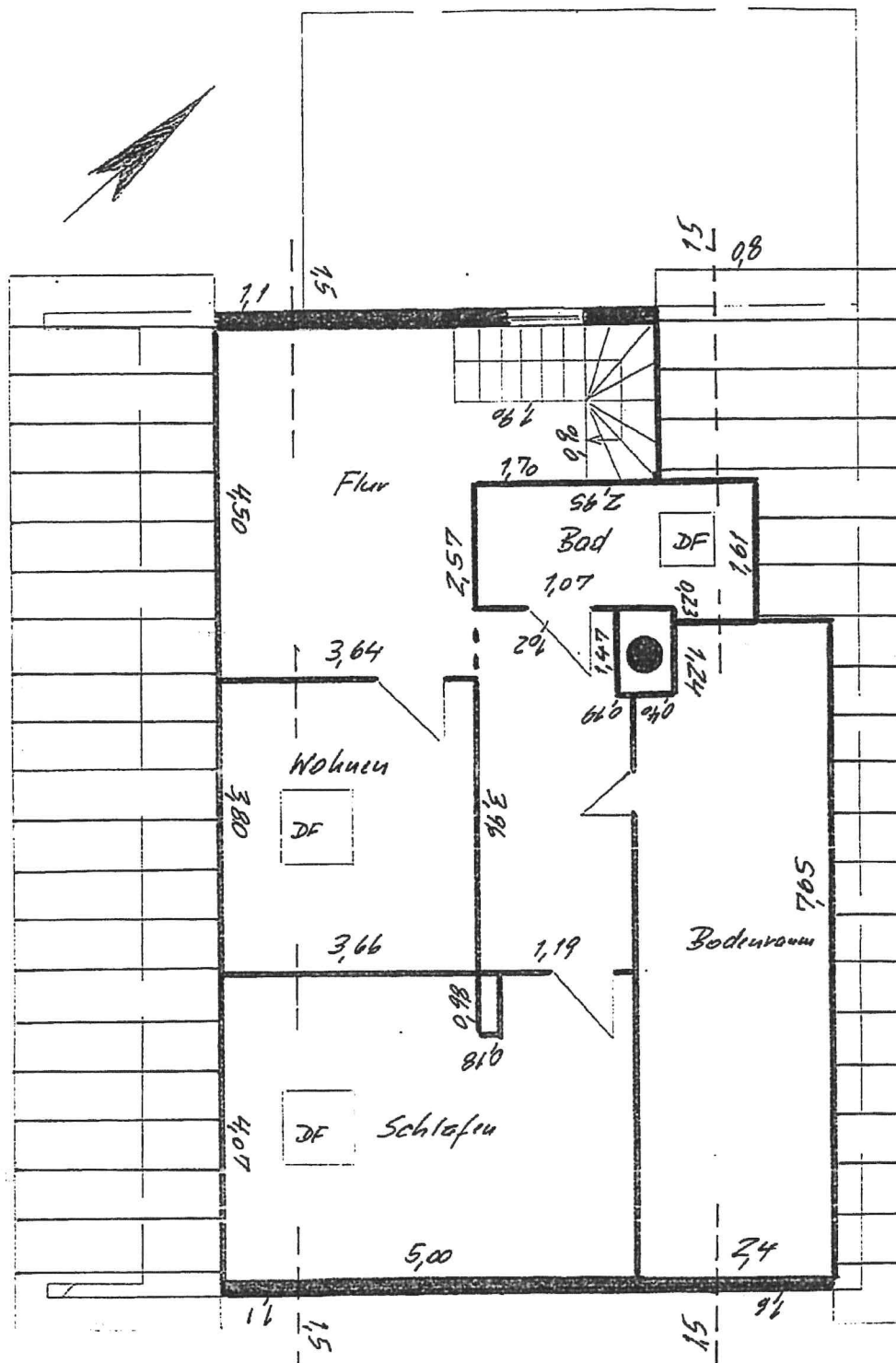
(Dachgeschossgrundriss – ohne Maßstab)
