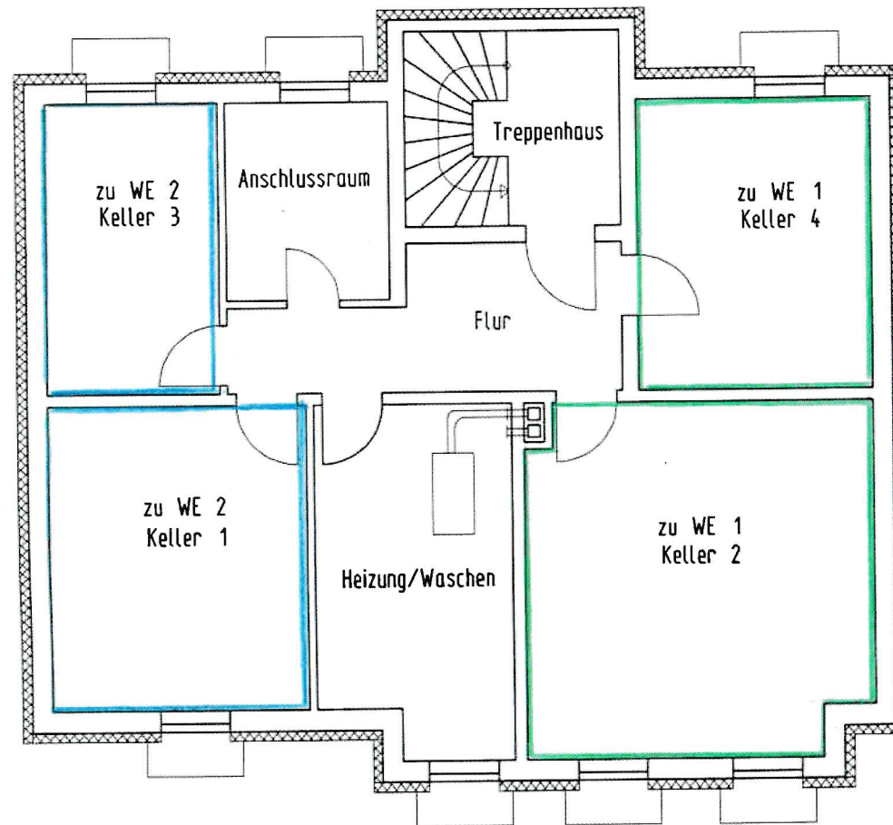
Kellergeschoss M1:100
