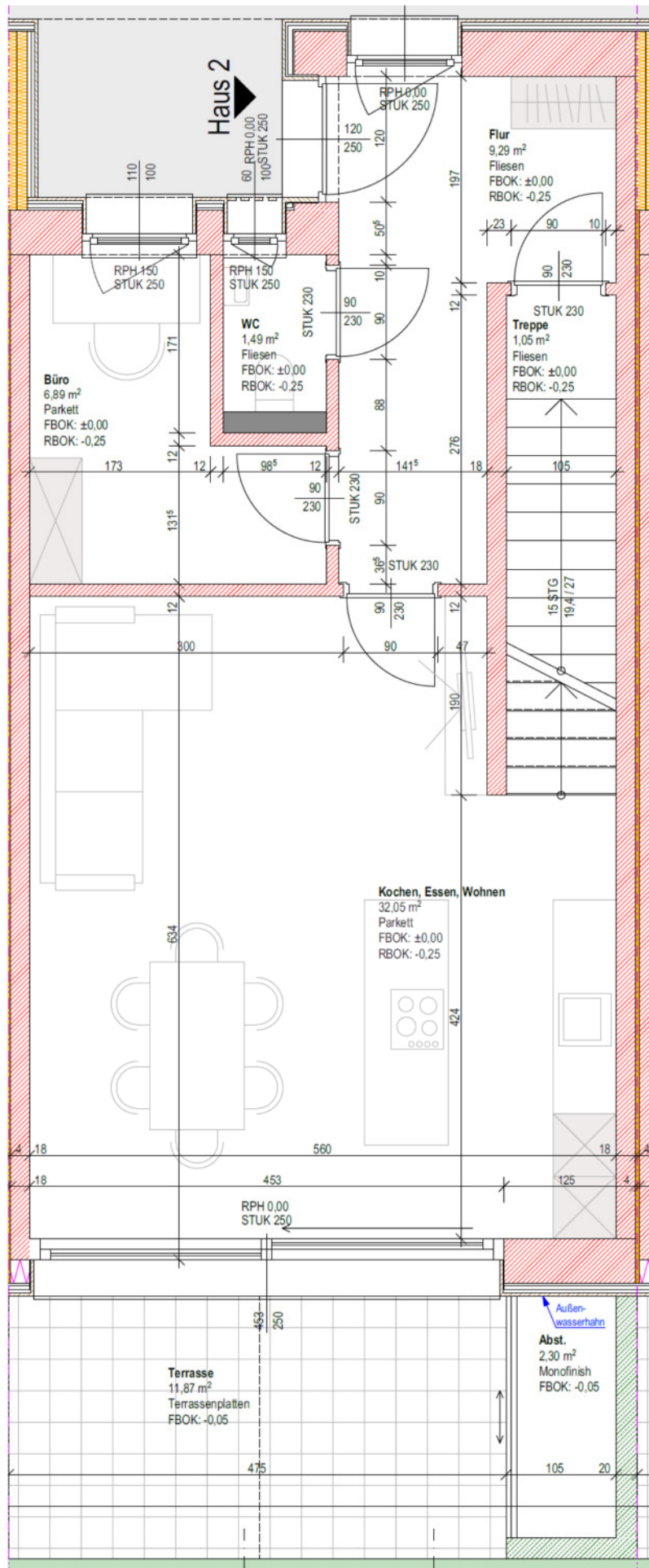
Erdgeschoß
