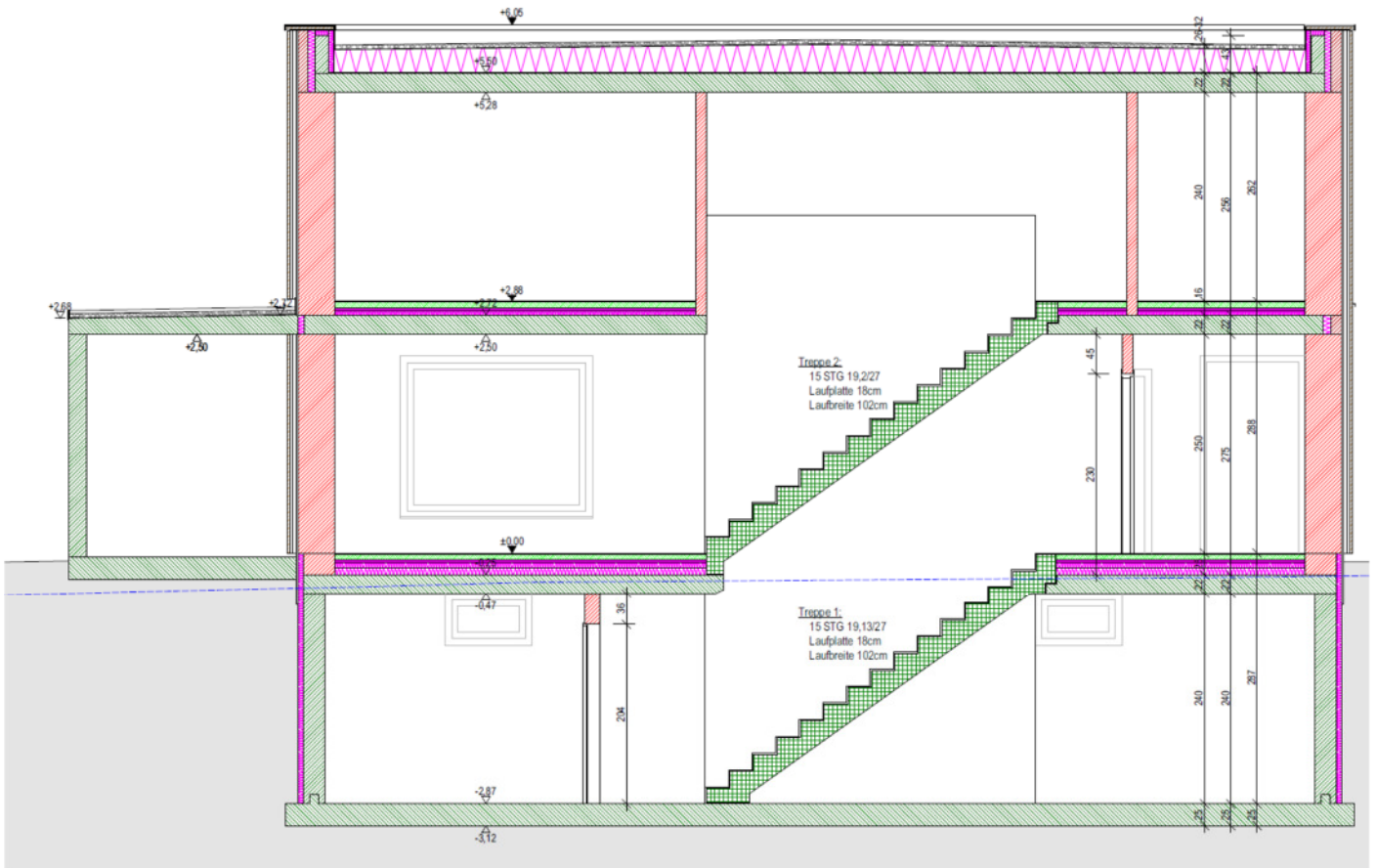
Schnitt
