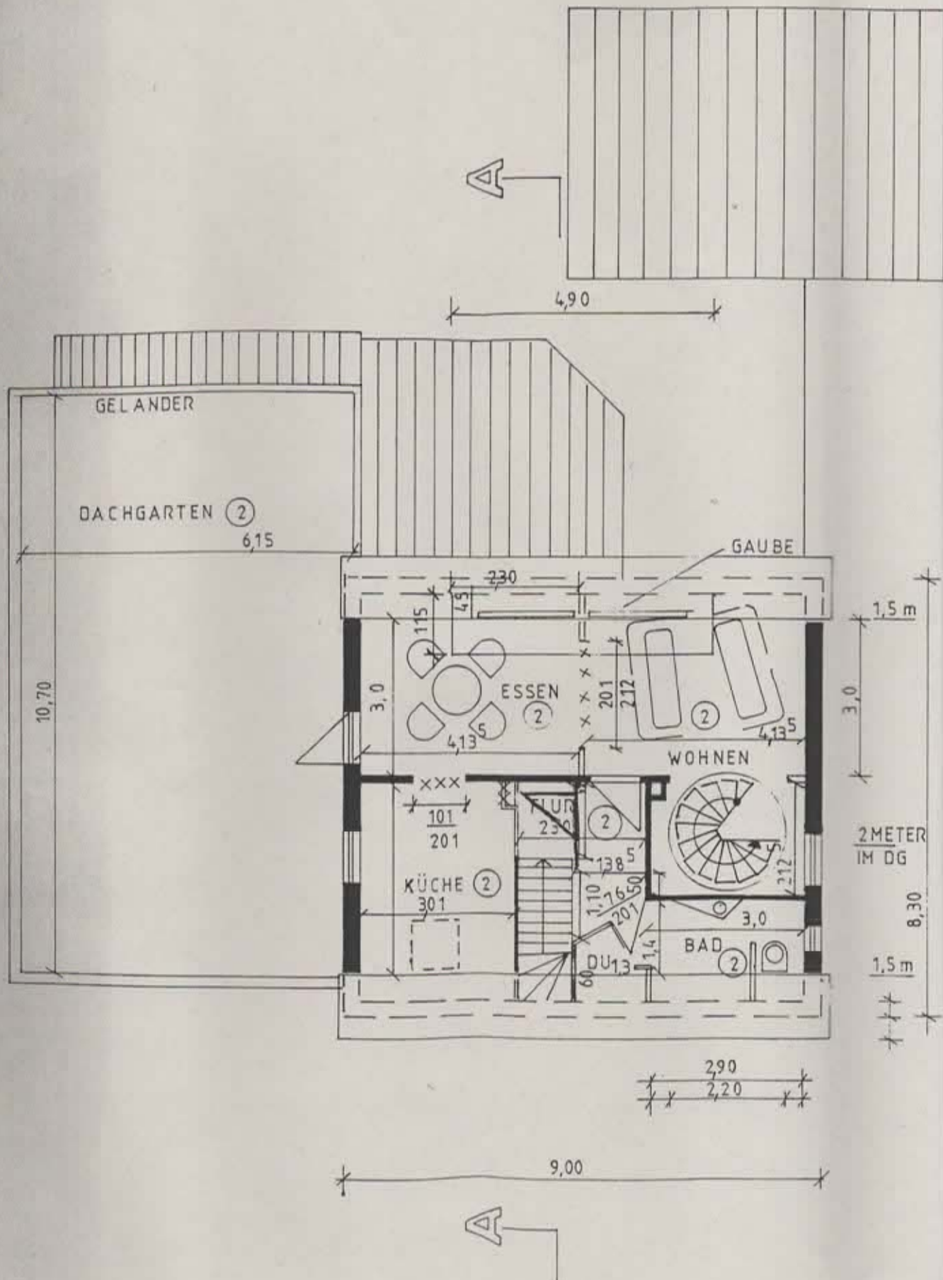
GRUNDRISS 10G
