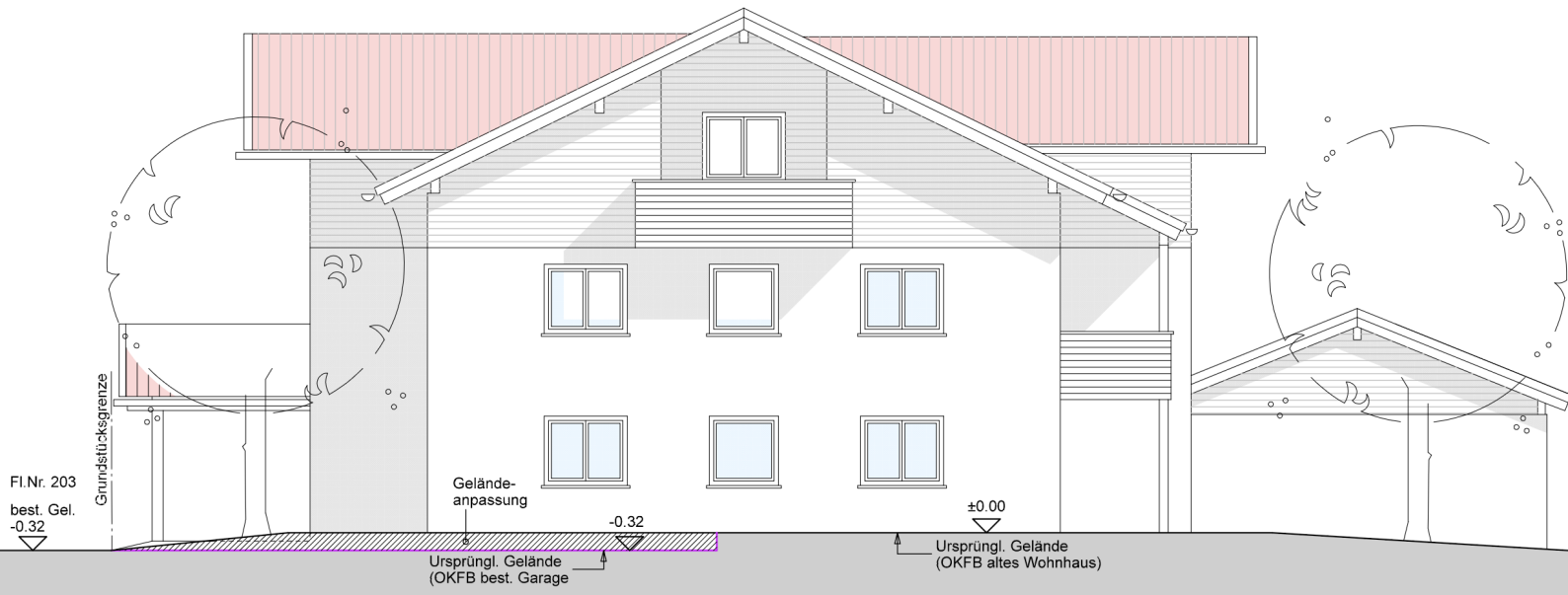
WESTANSICHT
