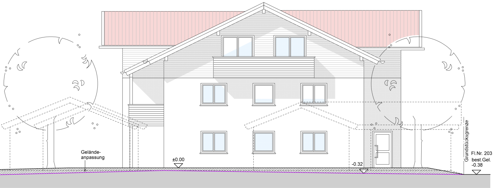
OSTANSICHT
