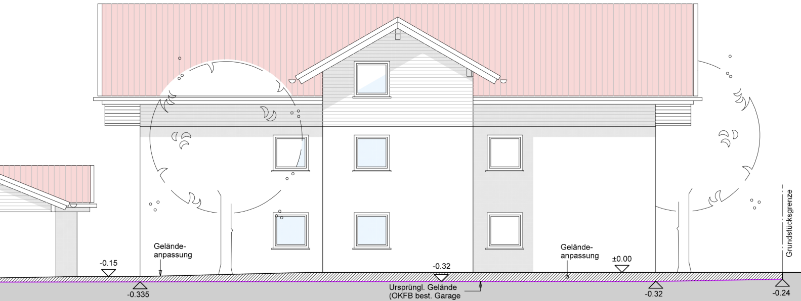
NORDANSICHT
