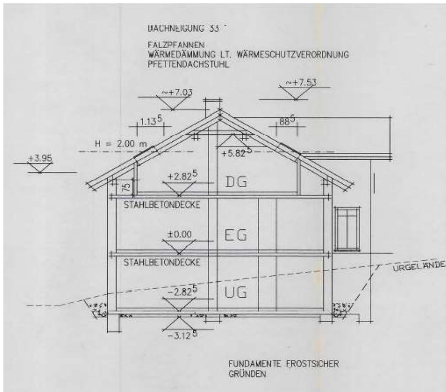
Schnitt Wohnhaus
