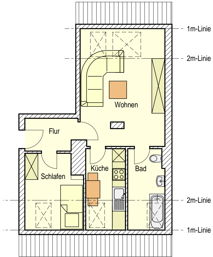
Typengrundriss
