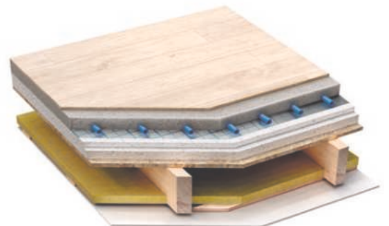
Schema Geschossdecke
