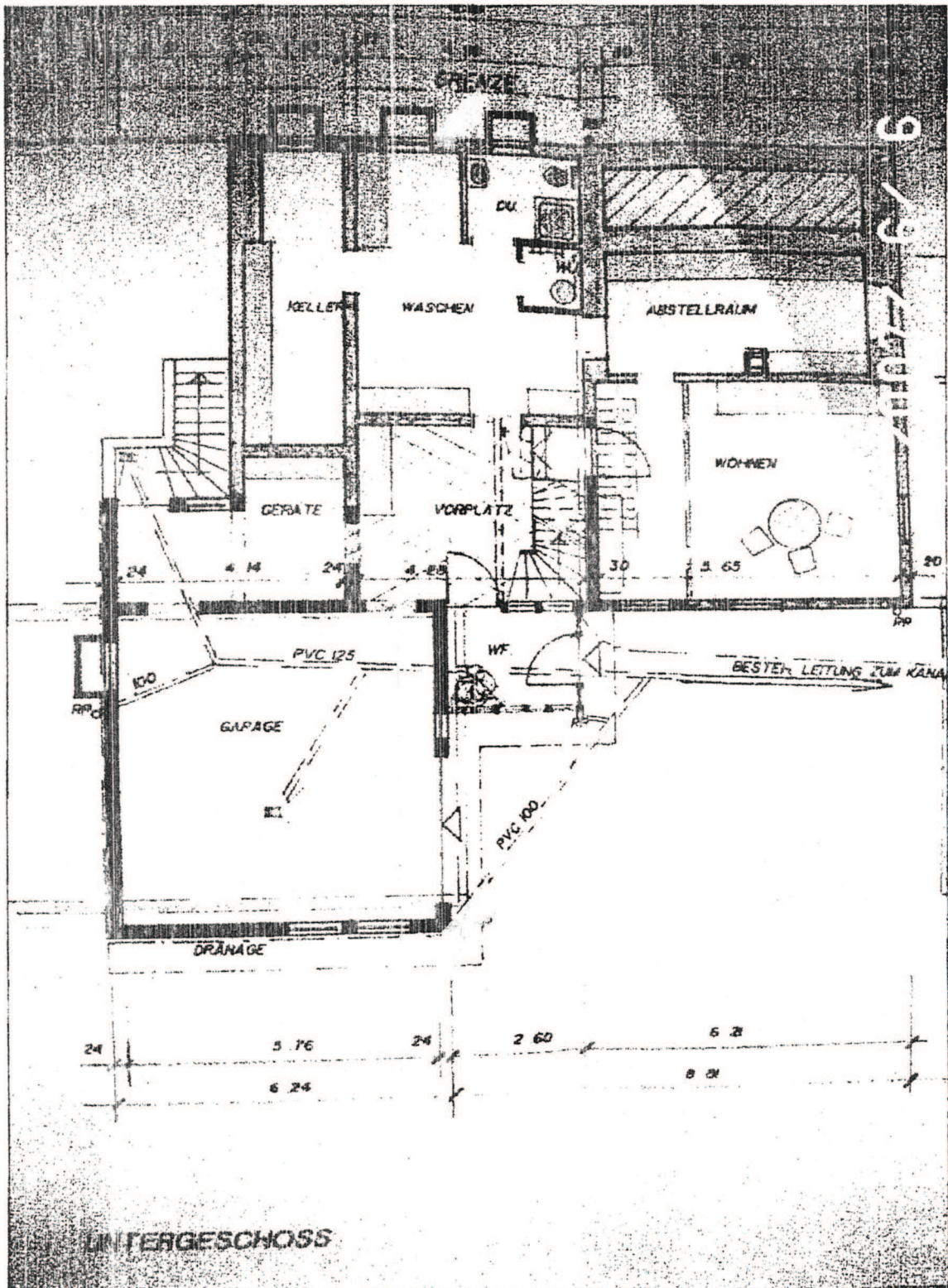
Grundriss UG im Maßstab 1:100
