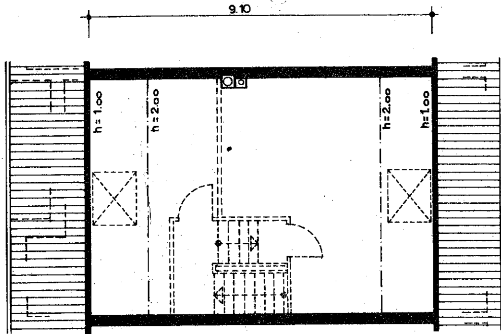
Dachgeschoss
