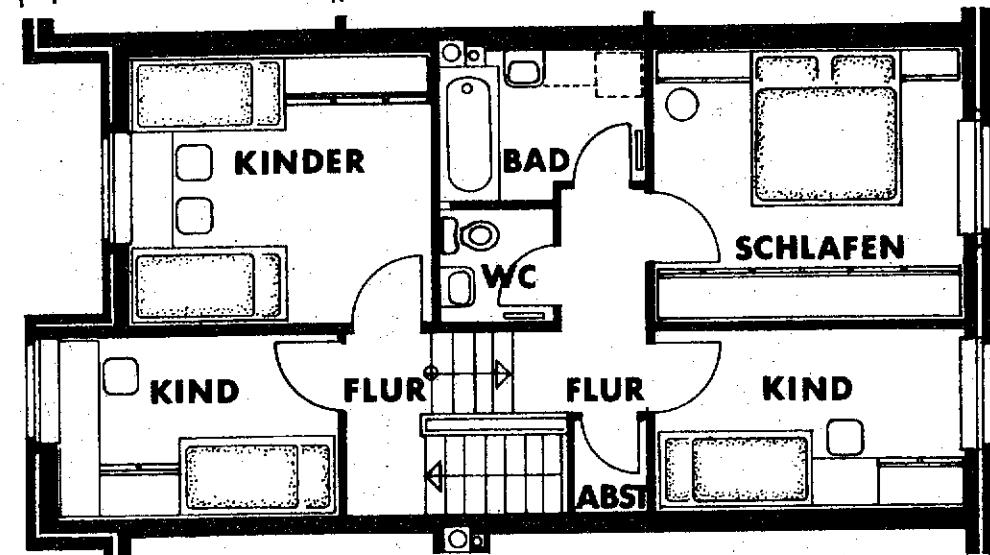
Obergeschoss
