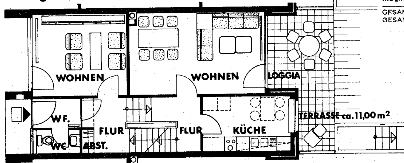
Erdgeschoss
