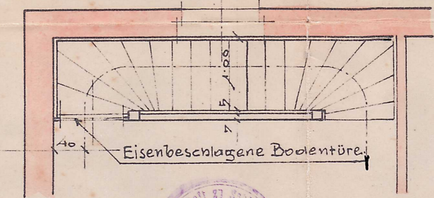
Stiege auf den Dachboden, aus Holz. 20 Stufenböden, à 15.75 hoch, Stufenbreite 27cm, am Stufenende 13cm.
