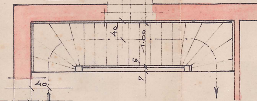
Stiege in den I Stock, aus Holz 21 Stufenböden, à 15.24 hoch, 25.25 breit, am Stufenende 13cm.
