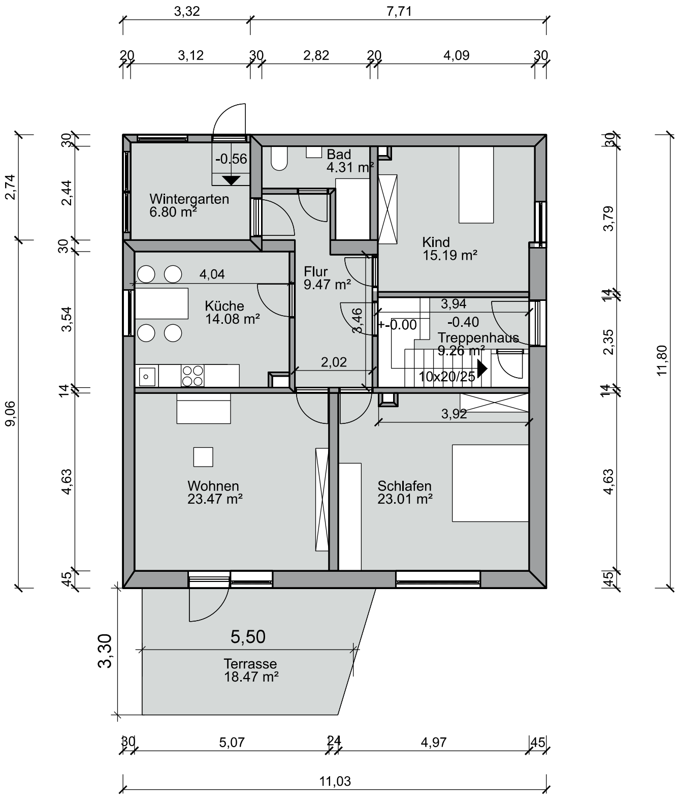
Grundriss Erdgeschoss
