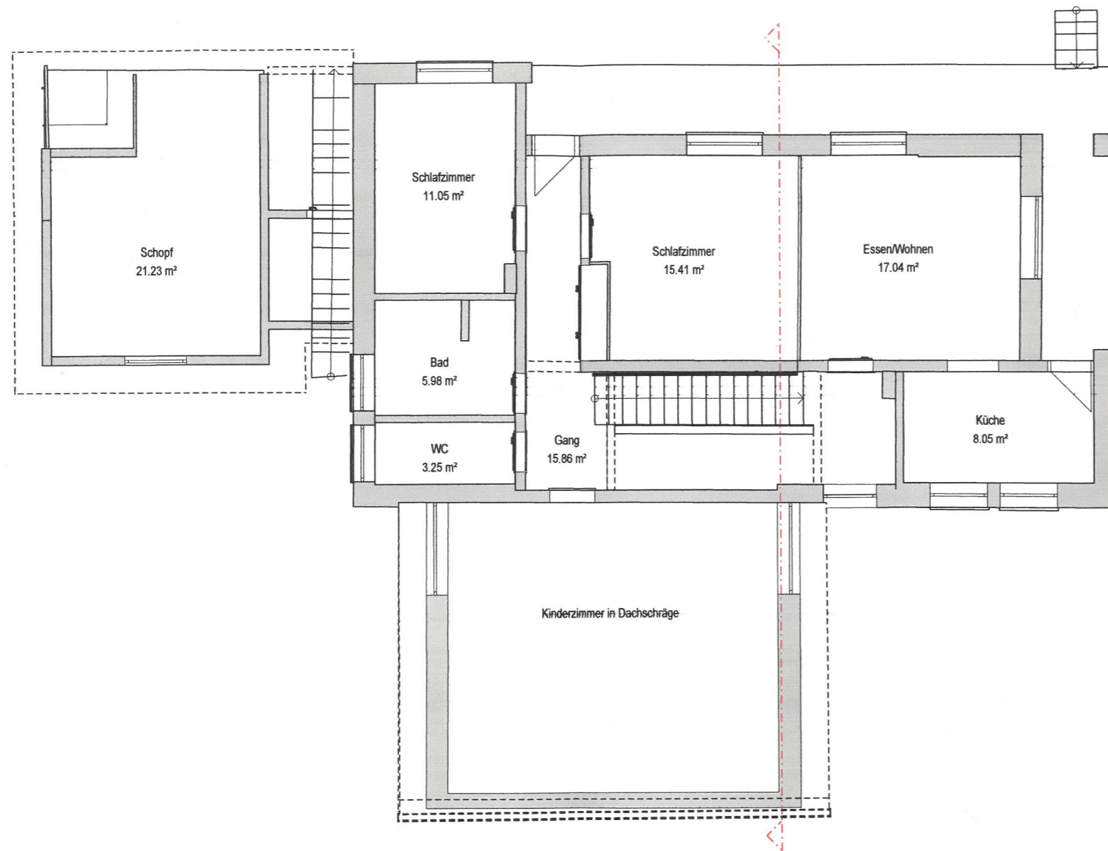
Grundriss Erdgeschoss
