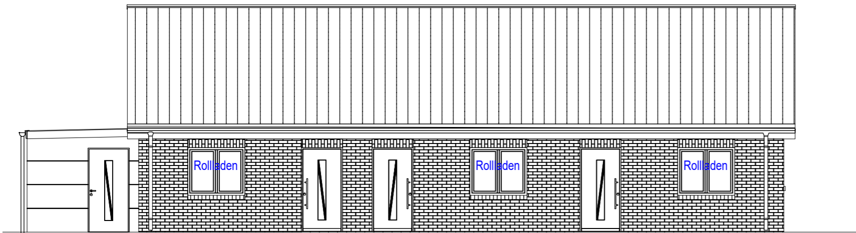
Ostansicht
