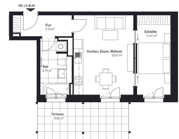
Grundriss
