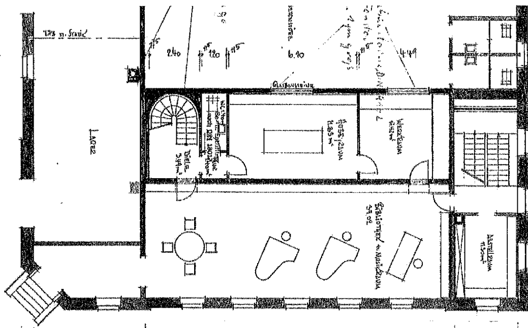
Wohnnutzung | Erdgeschoss
