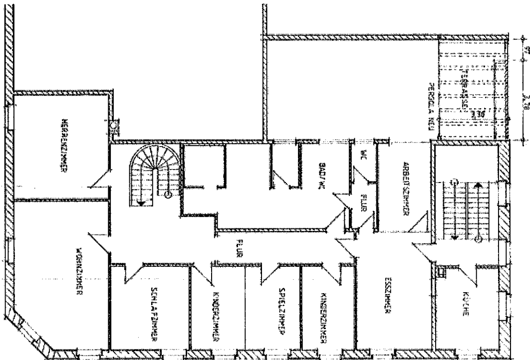
Wohnnutzung | Obergeschoss
