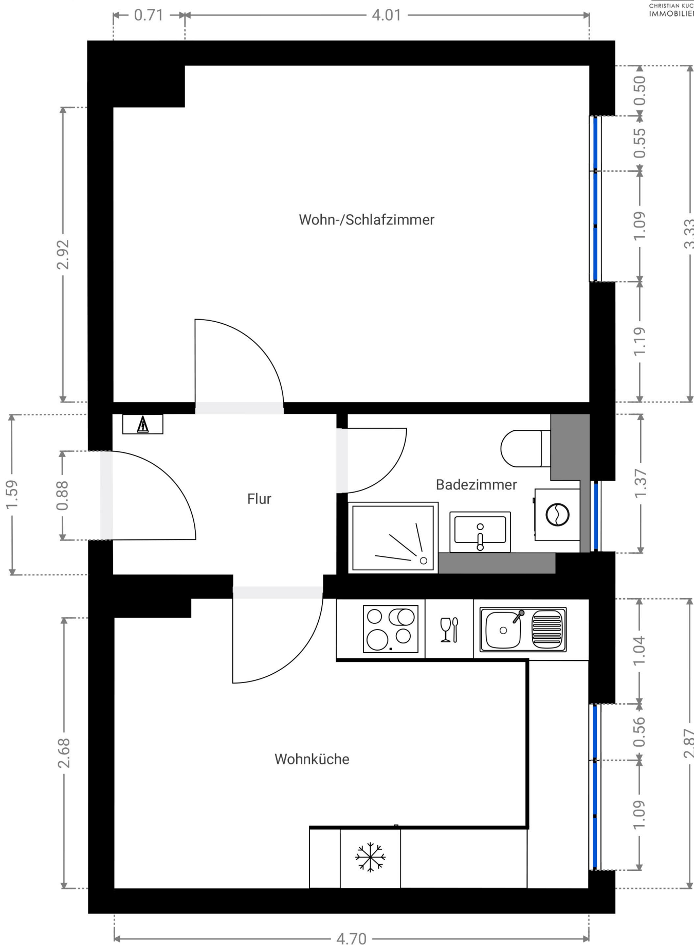
Grundriss WE04 Jägerstraße 27a
