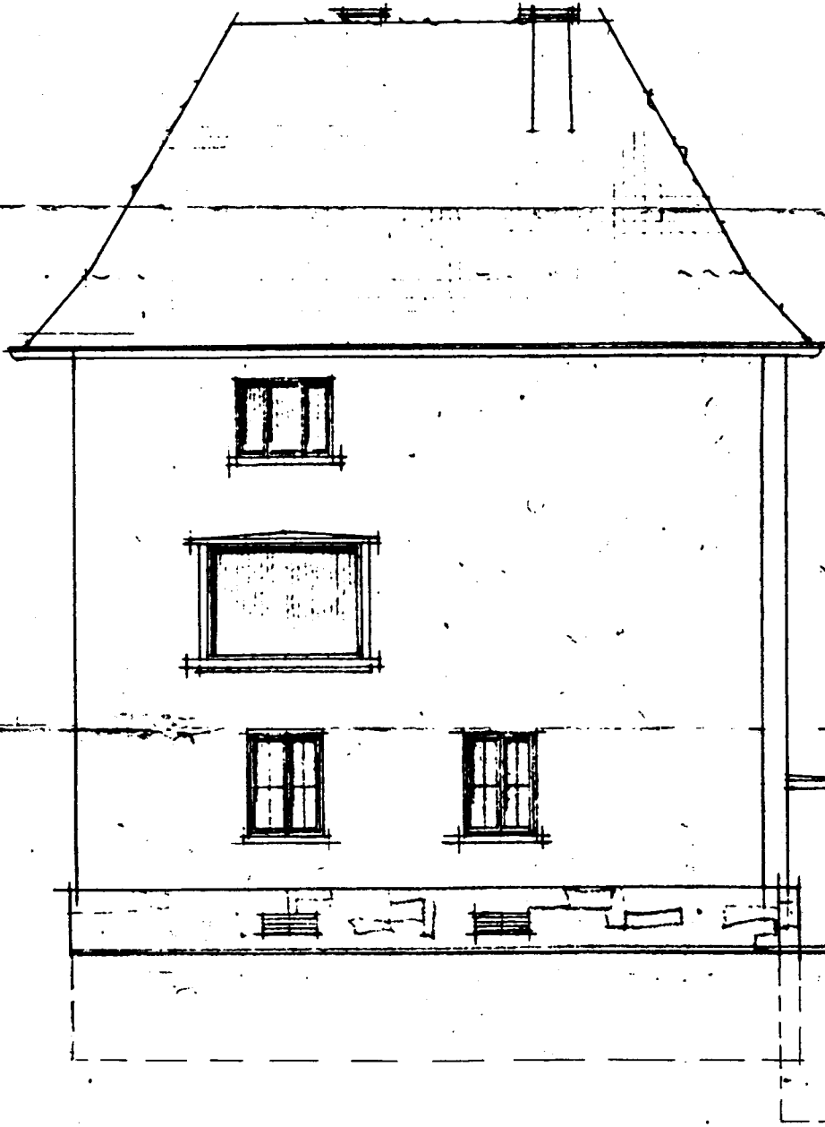
OSTANSICHT
