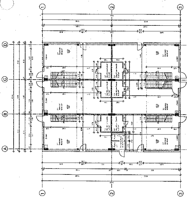
GEBÄUDE A - Erdgeschoss
