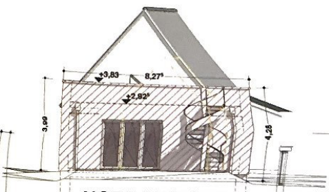
NORDANSICHT
