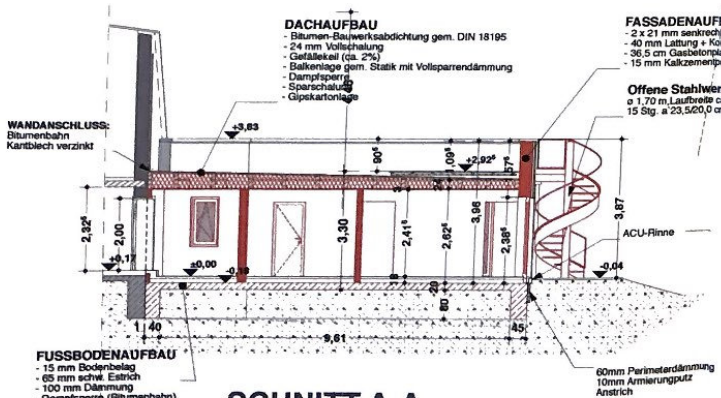
SCHNITT A-A
