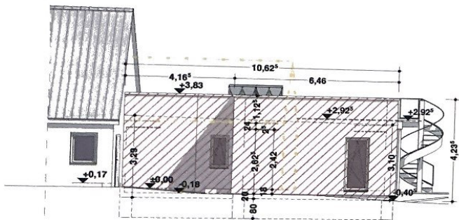
OSTANSICHT
