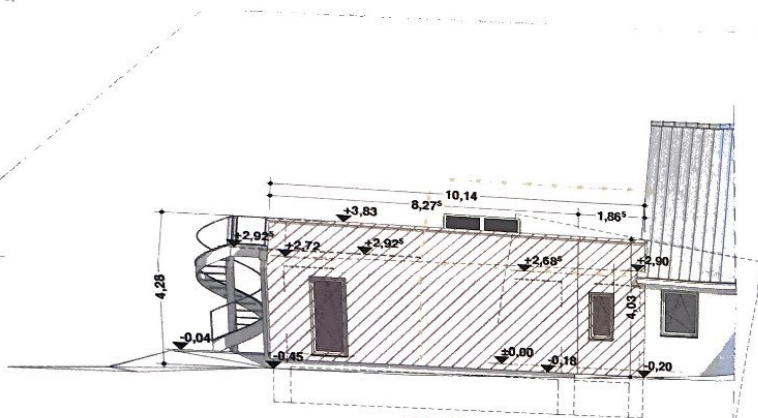
WESTANSICHT
