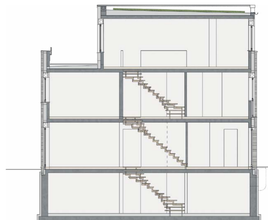
Exemplarischer Schnitt
