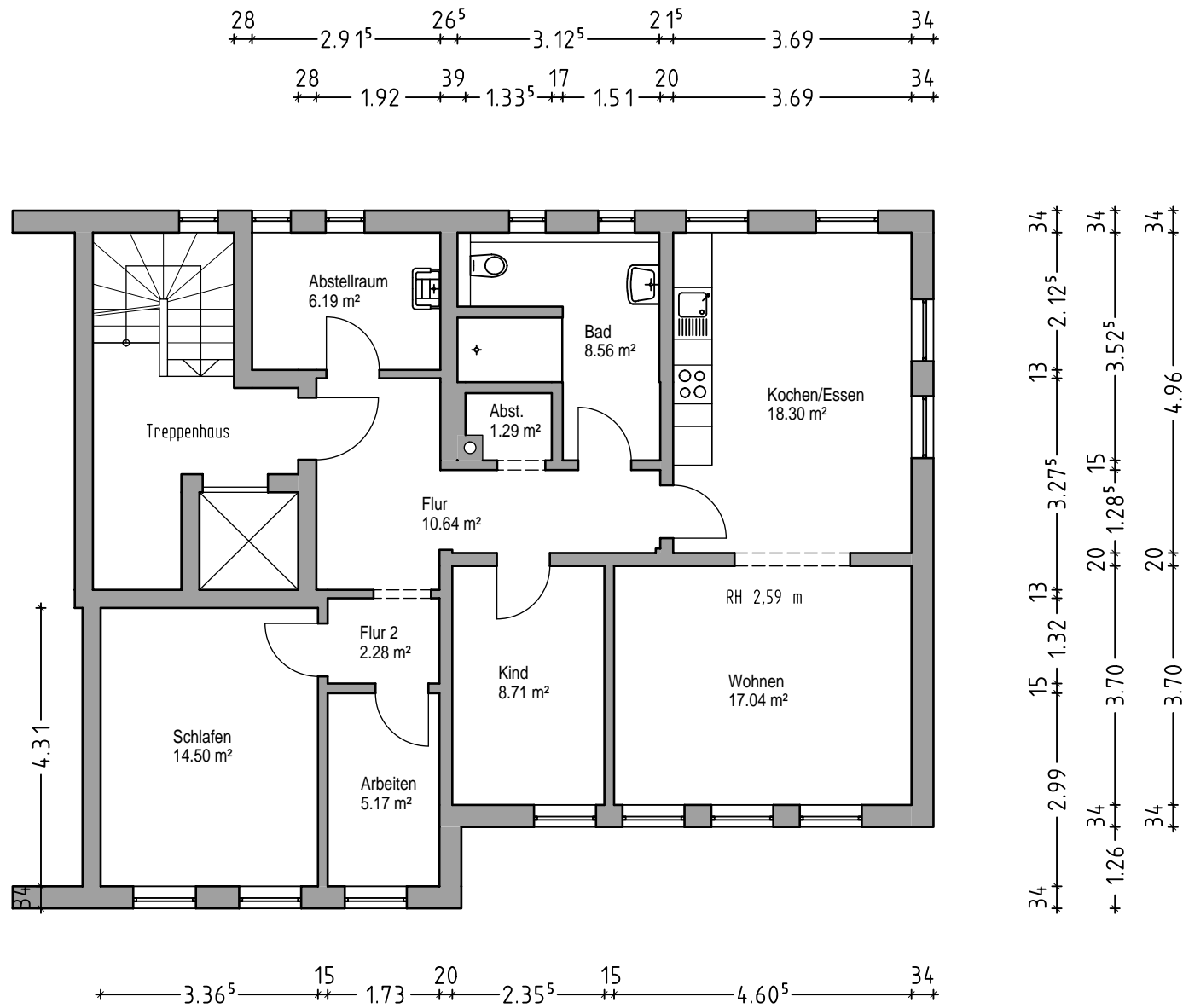
Bestandsplan M = 1:100 Stadtgraben 9 Beilngries 17.03.2026
