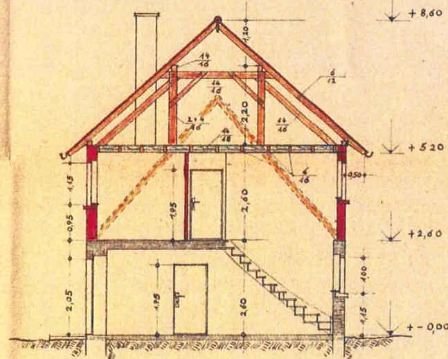
SCHNITT A - B
