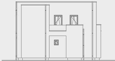
Ansicht Rechts
